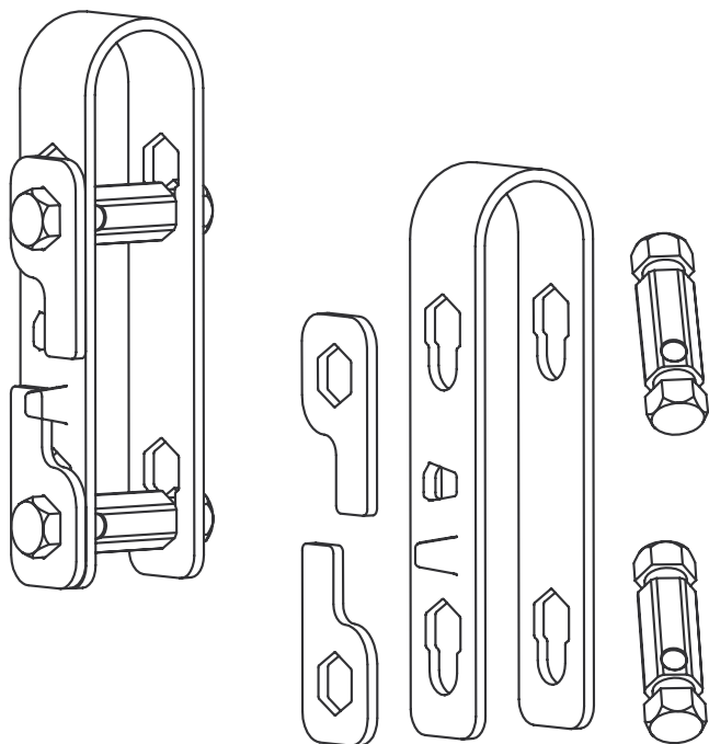
БОЛЬШОЙ НАТЯЖНОЙ АНКЕР
