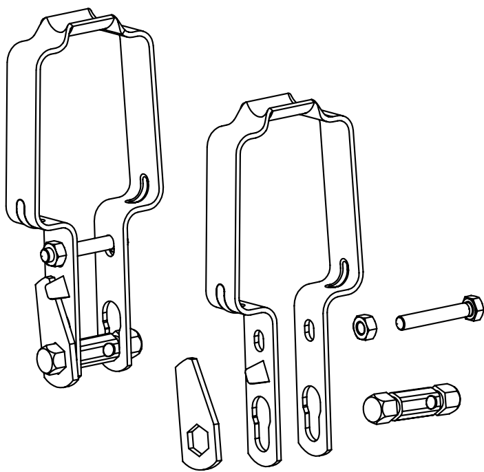
СКОБА ДЛЯ НАТЕЖЕНИЯ ПРОВОЛОКИ
