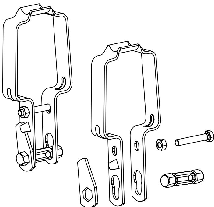
COLIER PENTRU ÎNTINDEREA FIRULUI
