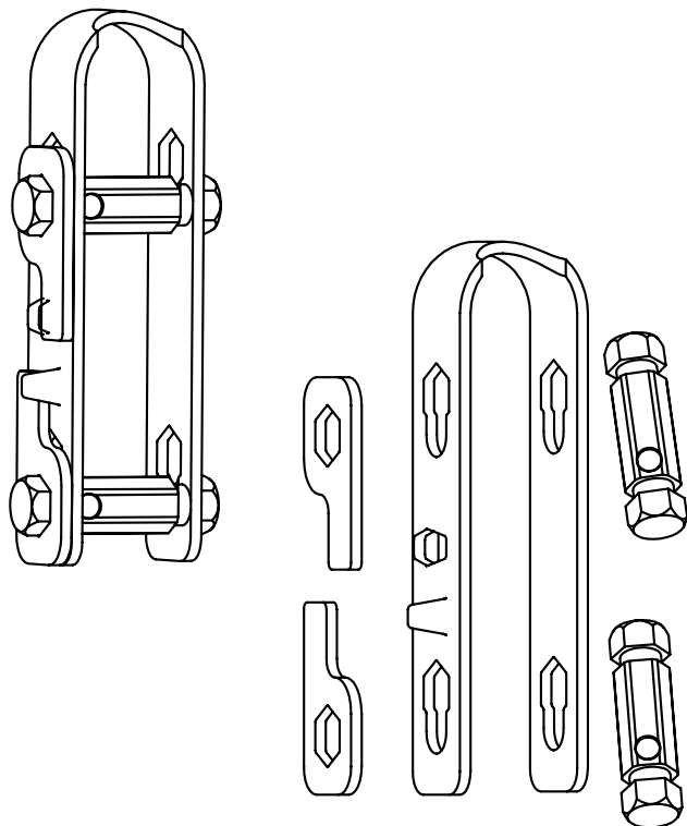
ÎNTINZĂTOR DE ANCORE MARI/SCURTE CU TEȘITURĂ
