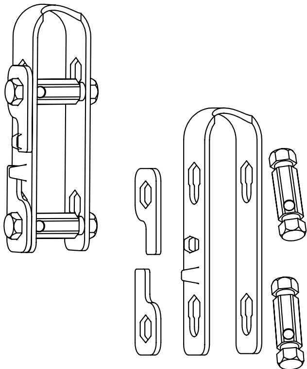
TENDIANCORA GRANDE CORTO CON SMUSSO
